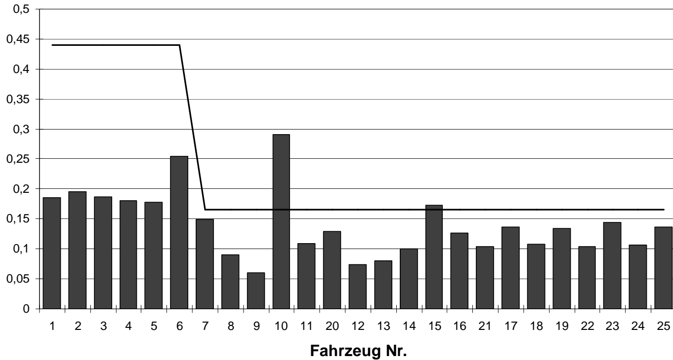
PM-Emissionen im 13-Stufen-Test in g/kWh
