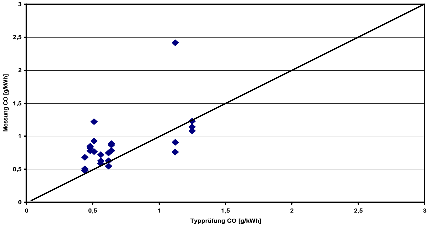
Vergleich der CO Emissionen Typprüfung/Feldüberwachung
