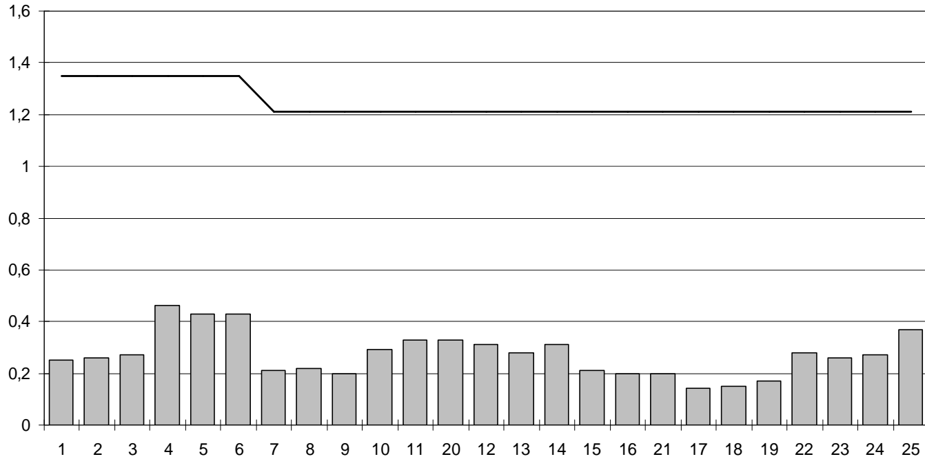
HC-Emissionen im 13-Stufen-Test in g/kWh
