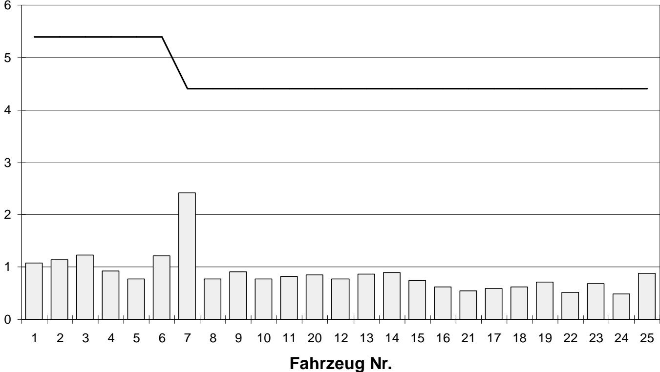
CO-Emissionen im 13-Stufen-Test in g/kWh
